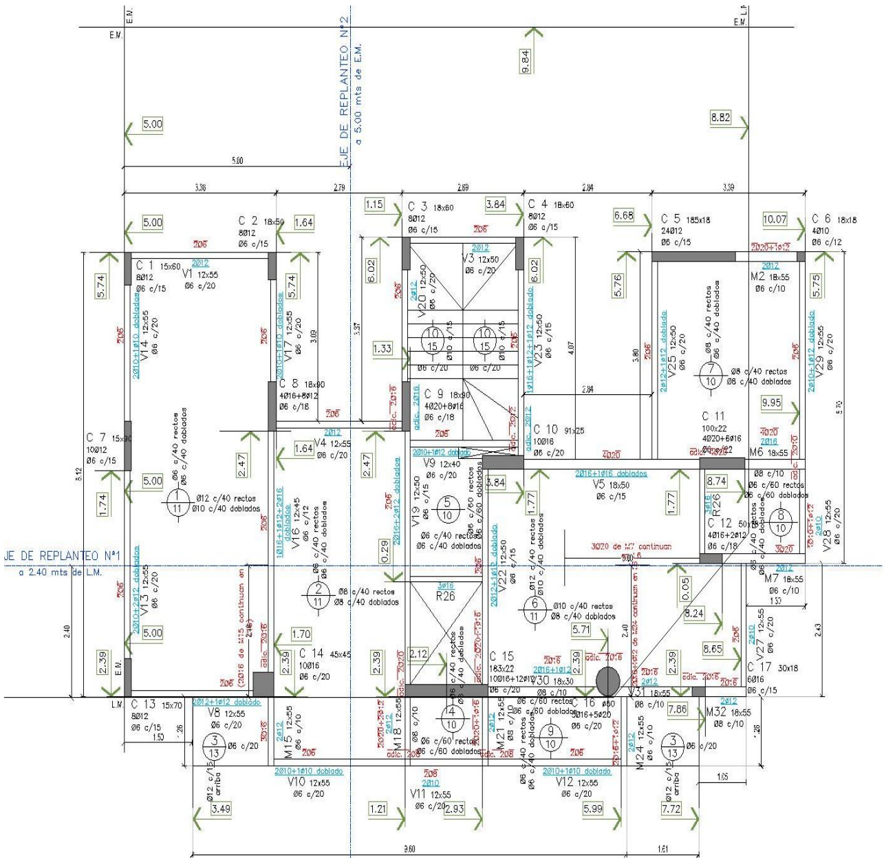
Imagen 11: Plano de estructura sobre planta TIPO.
