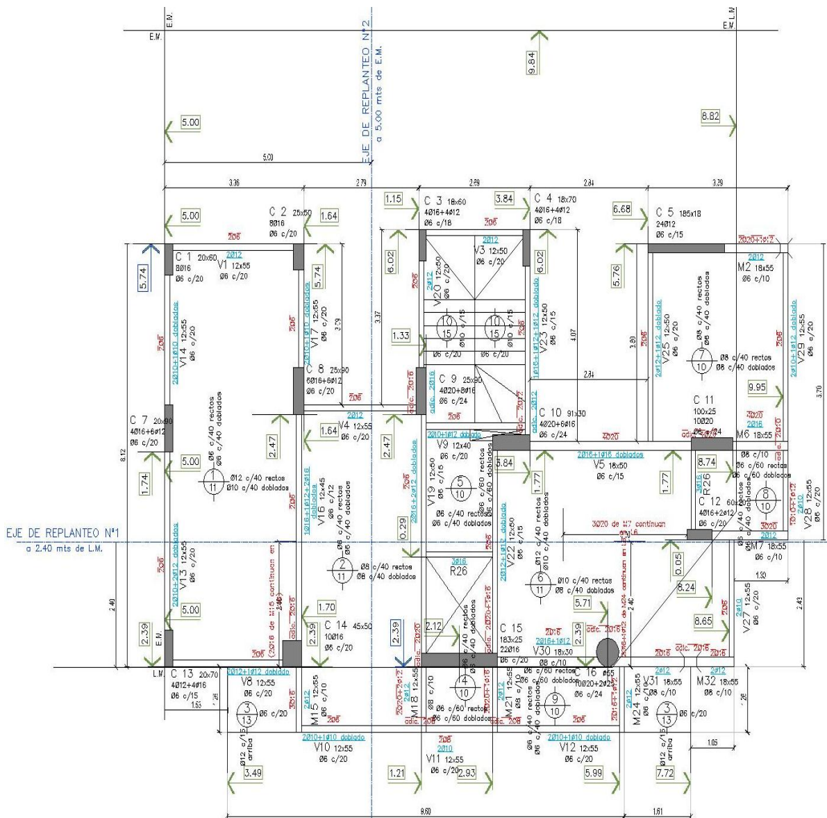
Imagen 10: Plano de estructura sobre planta baja.
